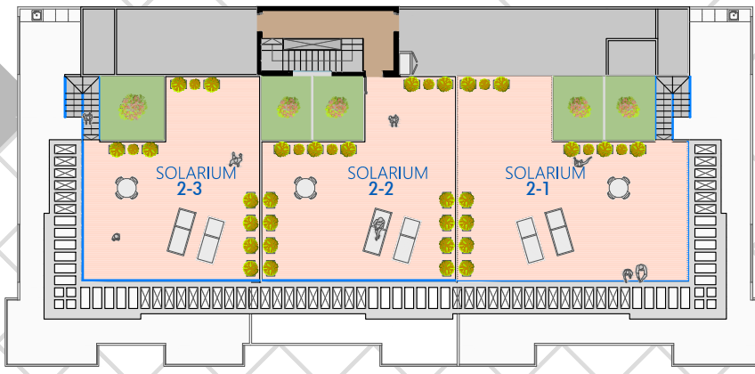
PLANTA CUBIERTA
